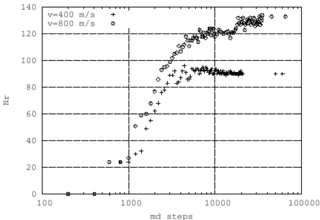
Fig.5. Variación del número de átomos en el cuello a 2 velocidades diferentes a T=300 K.
