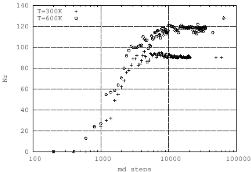
Fig.4 Variación del número de átomos en la región del cuello como función del tiempo a dos temperaturas diferentes y velocidad de colisión v = 400 m/s
