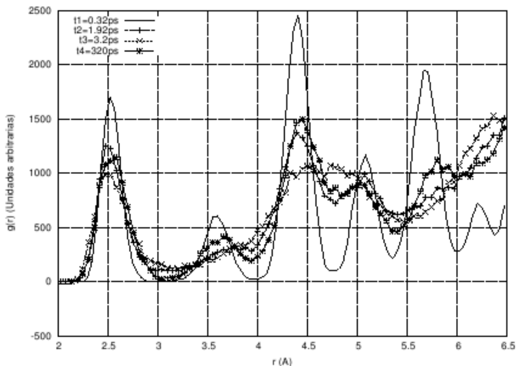
Fig.3: Funciones de distribución par en las diferentes etapas de la coalescencia de dos NP de cobre a temperatura 600 K.
