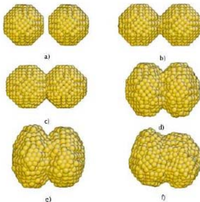
Fig.2: Evolución temporal del proceso de coalescencia a 300 K de dos NP de cobre con velocidad de impacto de 800 m/s: a) 0.32 ps, b) 0.96 ps, c) 1.60 ps, d) 2.88 ps, e) 3.84 ps, f) 8.64 ps. Para la visualización se utilizó el programa Atomeye [15]
